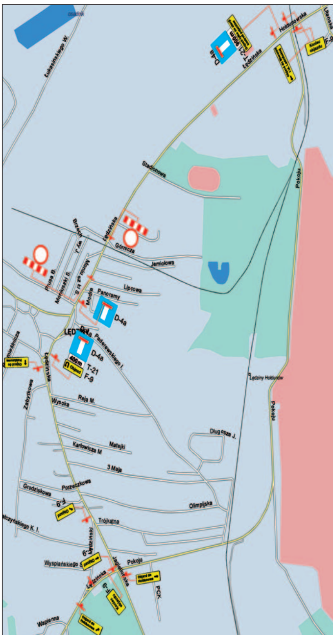
Rys. 1: Tymczasowa organizacja ruchu – zamknięcie odcinka drogi od ul. Lipcowej do stacji kontroli pojazdów.
