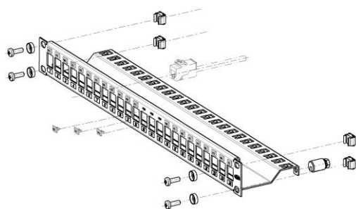
Rys.5 Panel 24 port ekranowany, kat.6
